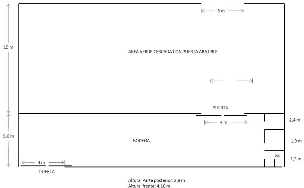
PLANO GENERAL DE LA BODEGA
